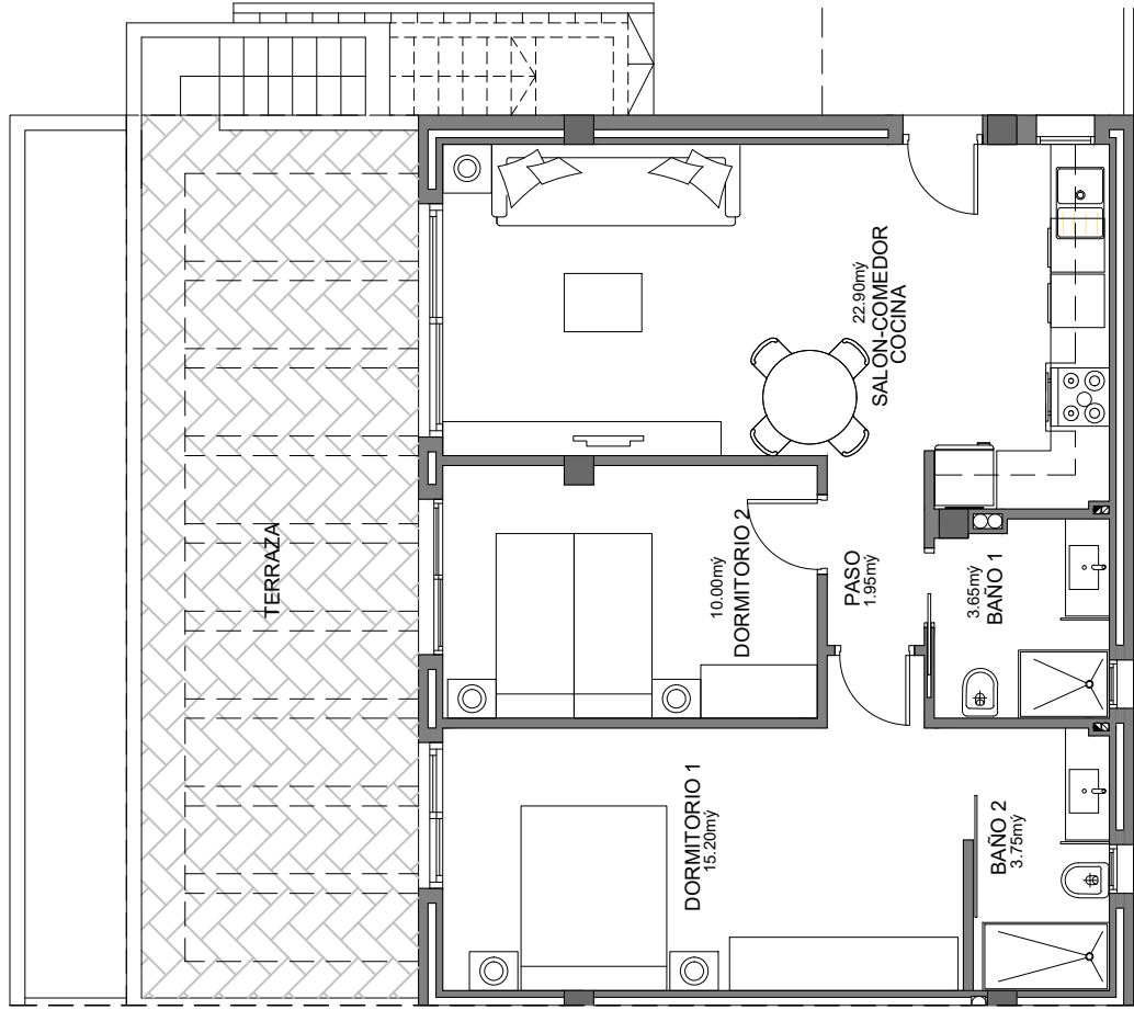
Planta Primera
