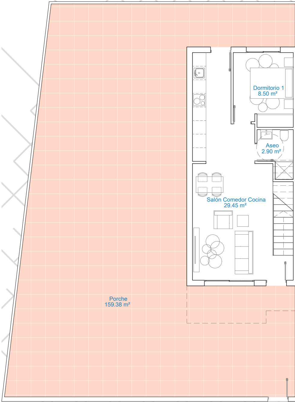
PLANTA BAJA
